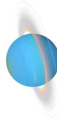
Uranus
